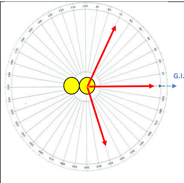
Appui moisé (ou jumelé) en angle
